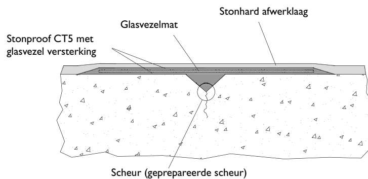
SCHEURBEHANDELING Stonproof CT5 met glasvezel versterking
