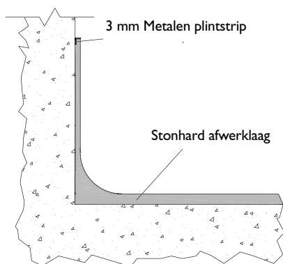
SANITAIRE PLINT MET PLINT STRIP
