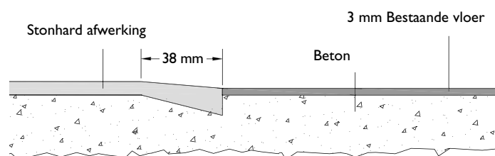
OVERGANG NAAR BESTAANDE VLOER
