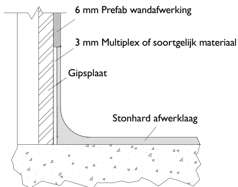
SANITAIRE PLINT met Prefab wandafwerking
