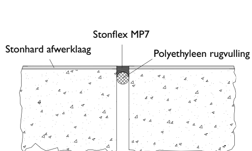
VOEGDETAIL / ISOLATIE VOEGDETAIL
