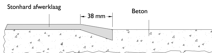
STANDAARD DWARSDOORSNEDE
