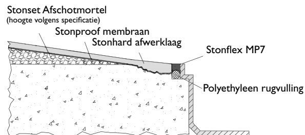
GOOT OVERGANG Prefab goot overgang met membraan
